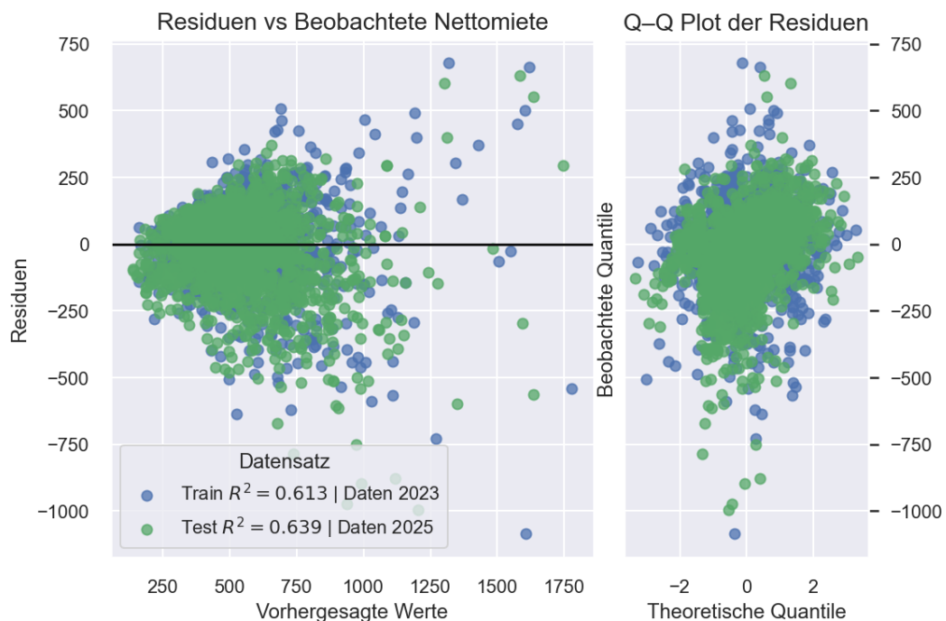
Abbildung 4: Residuen-Diagnostik eines linearen Regressionsmodells. Links ist der Residuen-gegen-Vorhersage-Plot für Trainings- (Daten 2023) und Testdaten (Daten 2025) dargestellt; die angegebenen R^2 -Werte quantifizieren die Modellgüte auf beiden Datensätzen. Rechts zeigt der Q-Q-Plot die Verteilung der standardisierten Residuen im Vergleich zu einer Normalverteilung.
